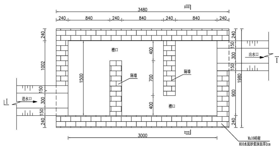
图 5-3 沉沙池平面图
