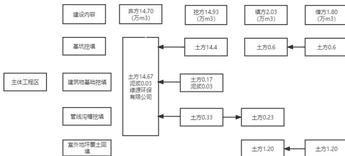
图 2-2 土石方流向框图 (单位: \text{万 m}^3 )
