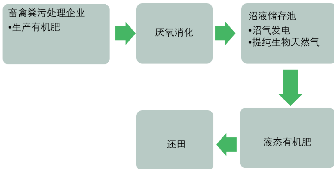
图 6-15 粪水肥料化利用模式流程图
