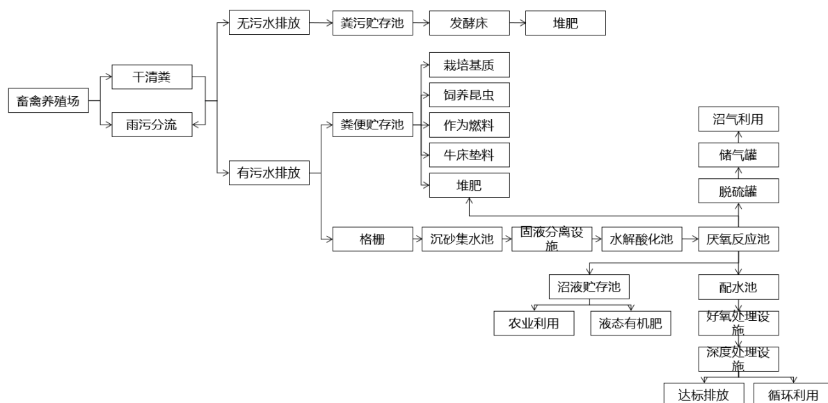
图 6-13 畜禽养殖粪污处理利用工艺流程图
