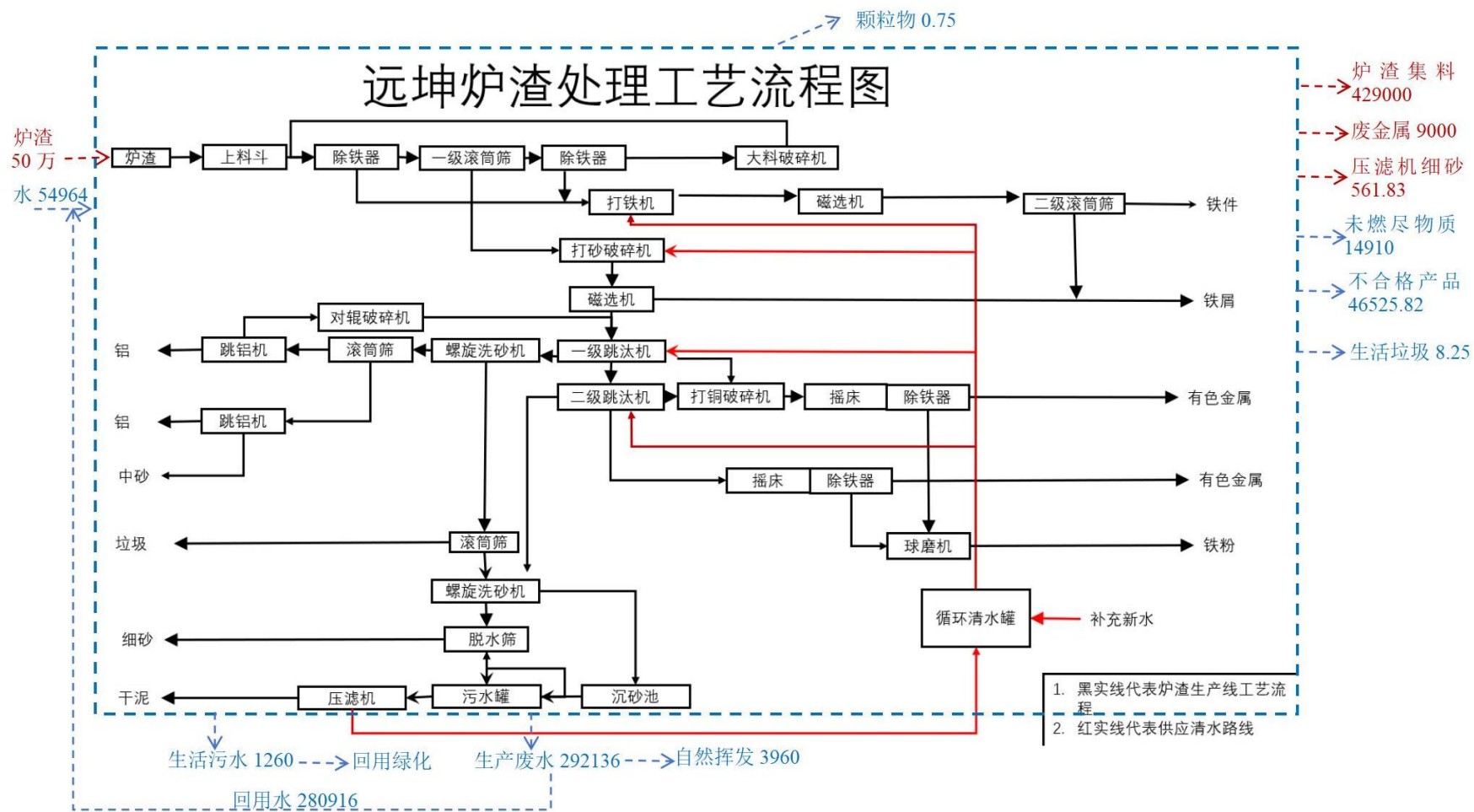
图 2-5 项目物料平衡示意图
