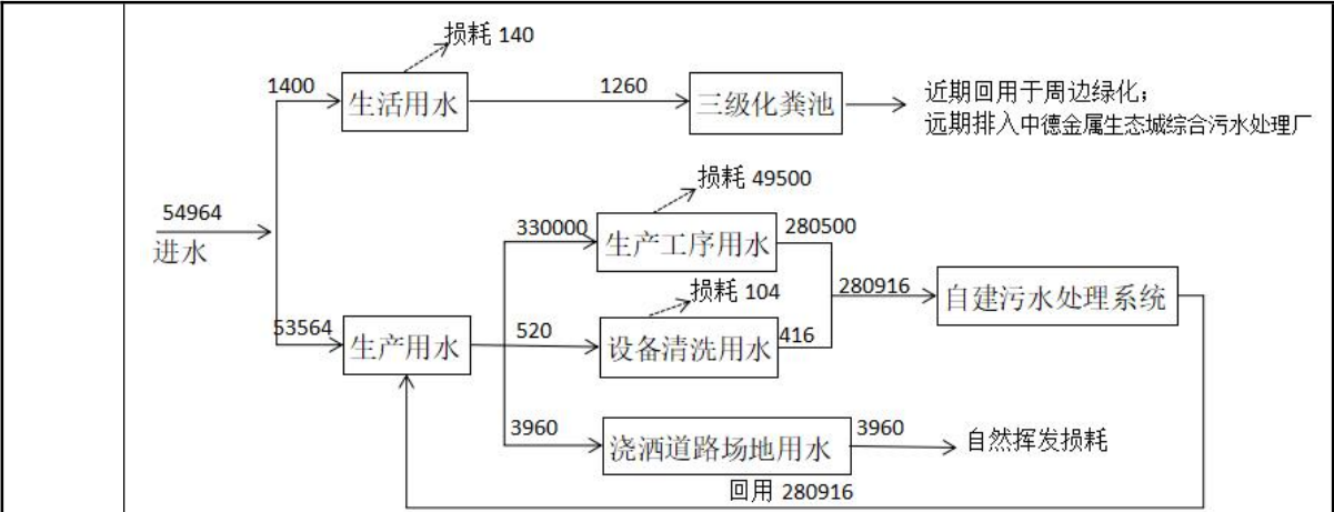
图 2-1 厂区水平衡图 (t/a)
