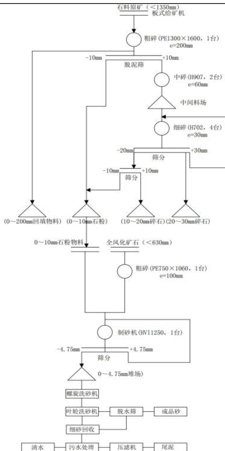
图 2-1 矿山加工工艺流程图
