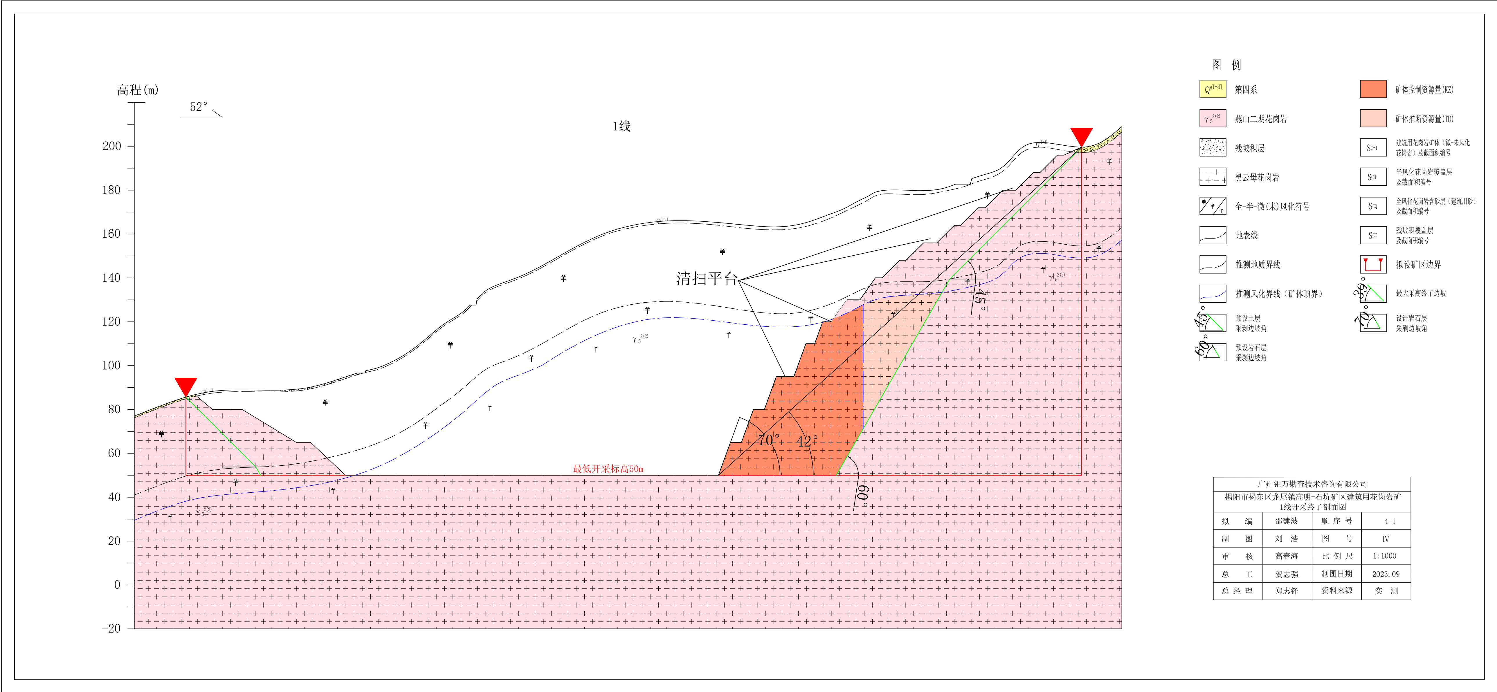
揭阳市揭东区龙尾镇高明-石坑矿区建筑用花岗岩矿1线开采终了剖面图 比例尺1: 1000
