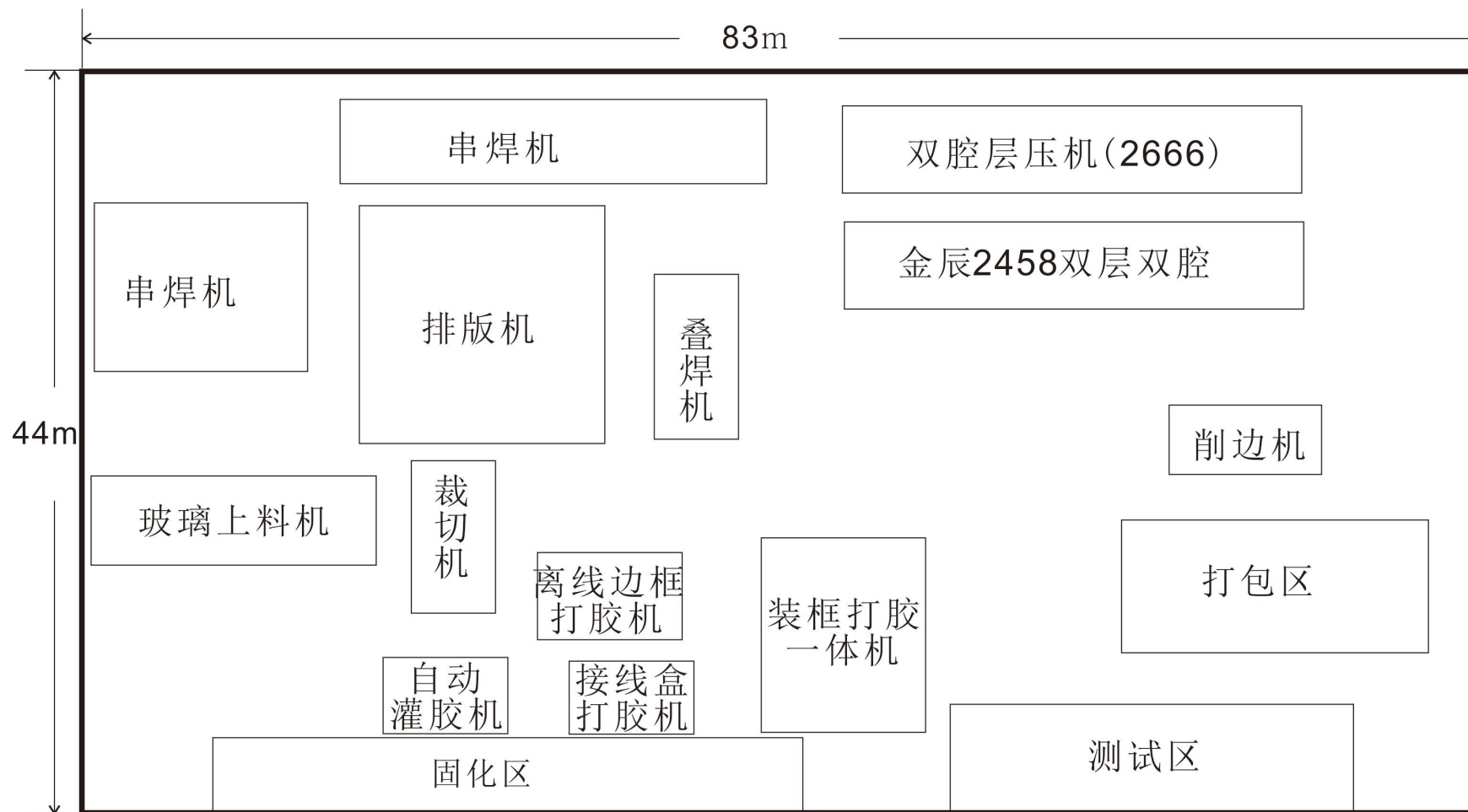
附图 3-1 车间平面布置图
