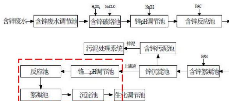
图 2-5 含锌废水物化处理工艺流程图
