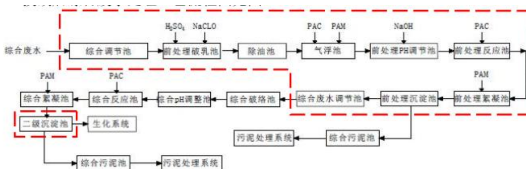
图 2-7 综合废水物化处理工艺流程图
