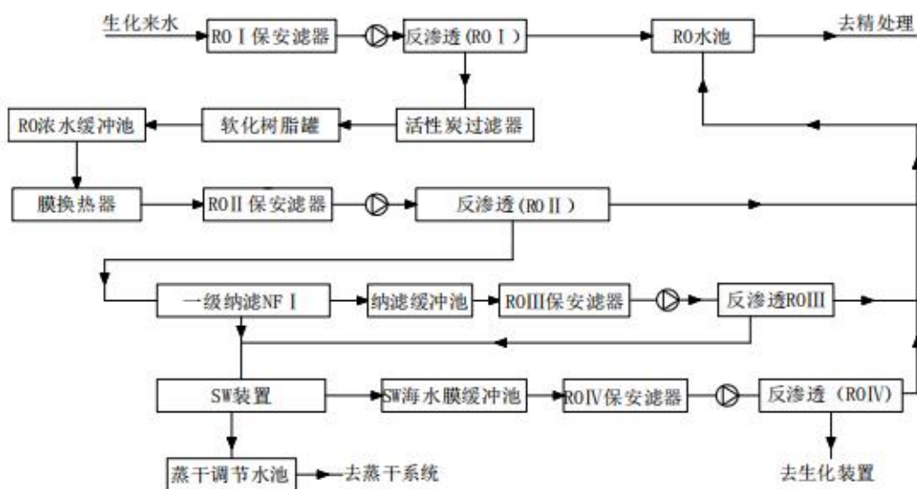
图 2-10 蒸干处理系统工艺流程图
