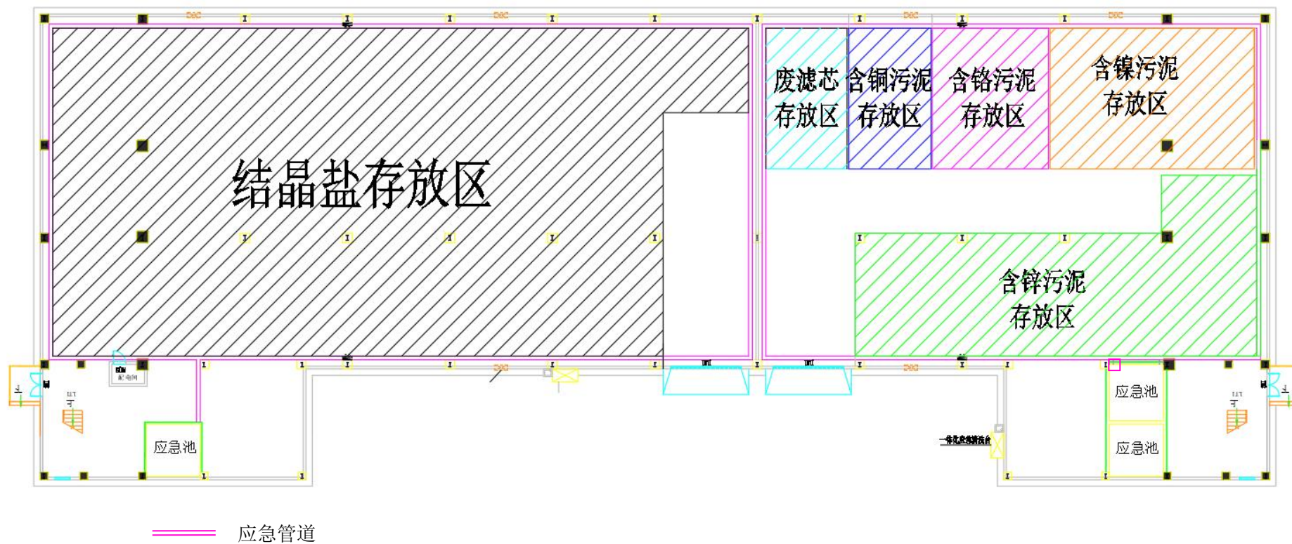
附图五 项目平面布置图
