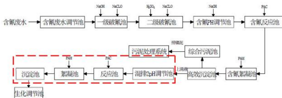
图 2-4 含氰废水物化处理工艺流程图
