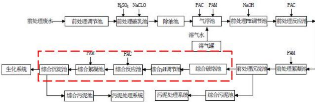
图 2-3 前处理废水物化处理工艺流程图
