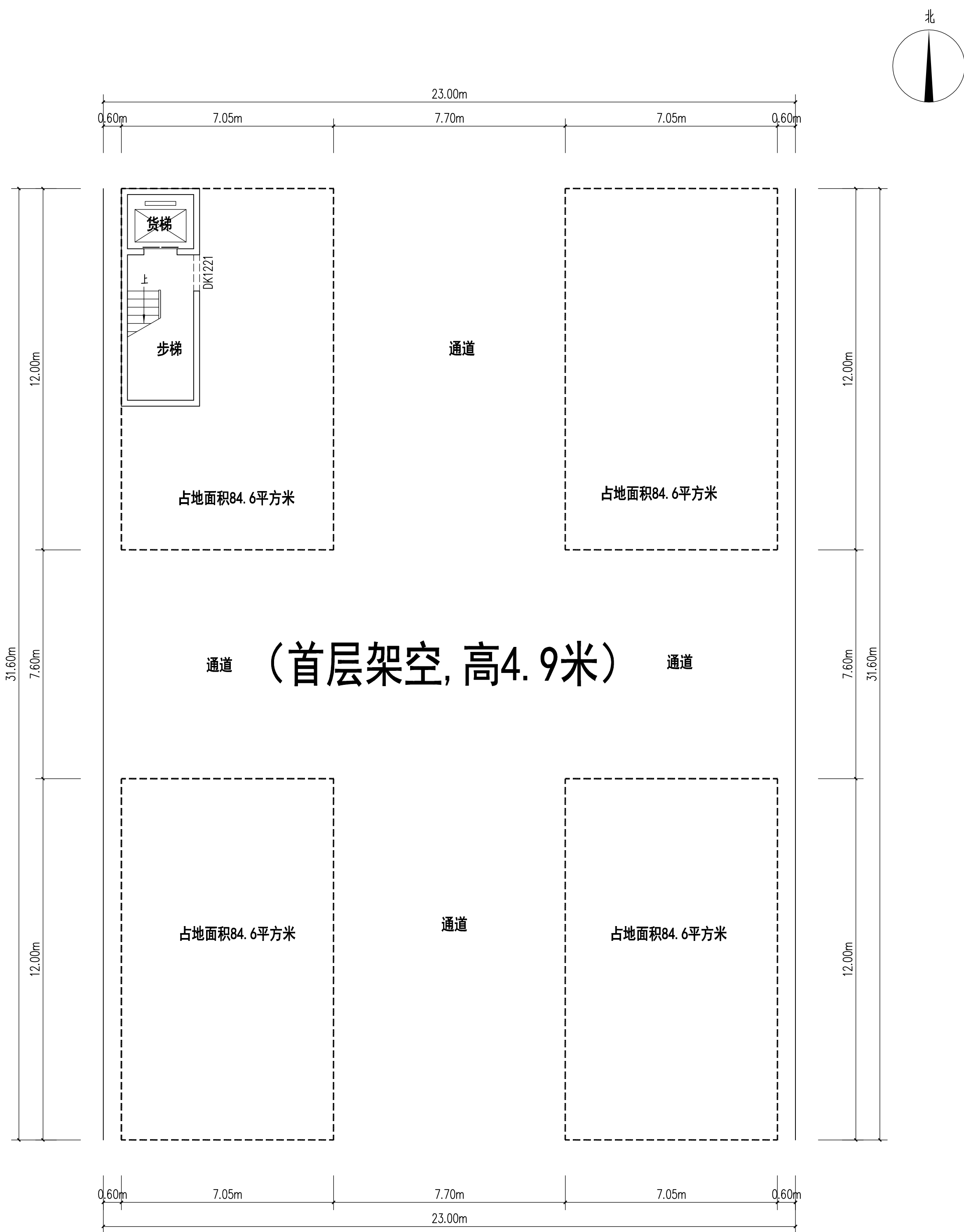
首层平面图 1:100
