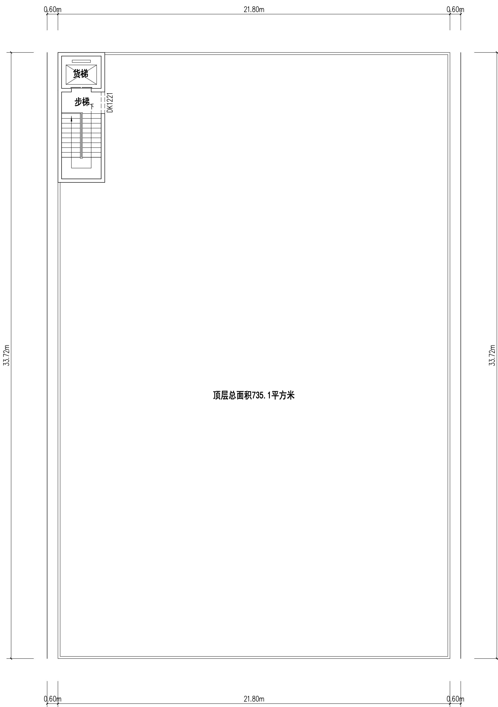
顶层平面图 1:100
