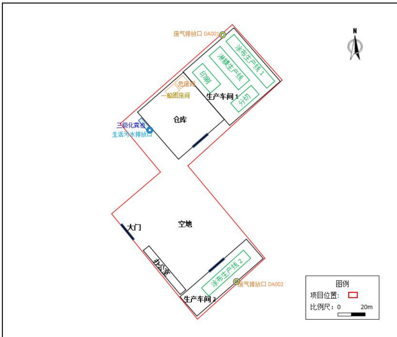
附图 3 项目平面布局图
