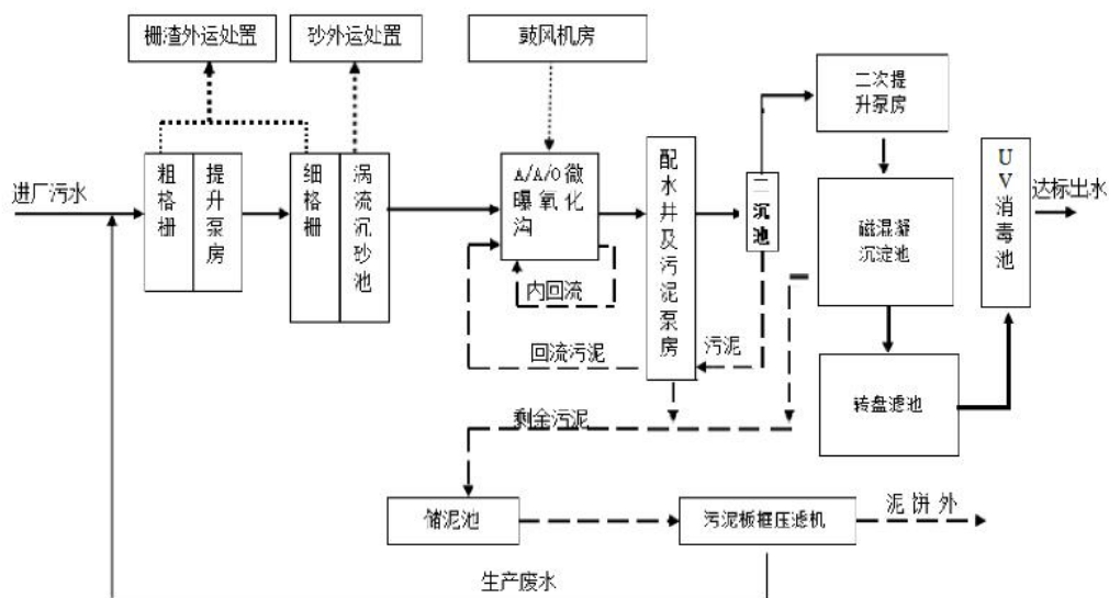
图 4-1 污水处理工艺流程图
