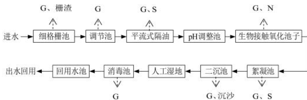
图中：G--废气；S--污泥；N--噪声；→污水
