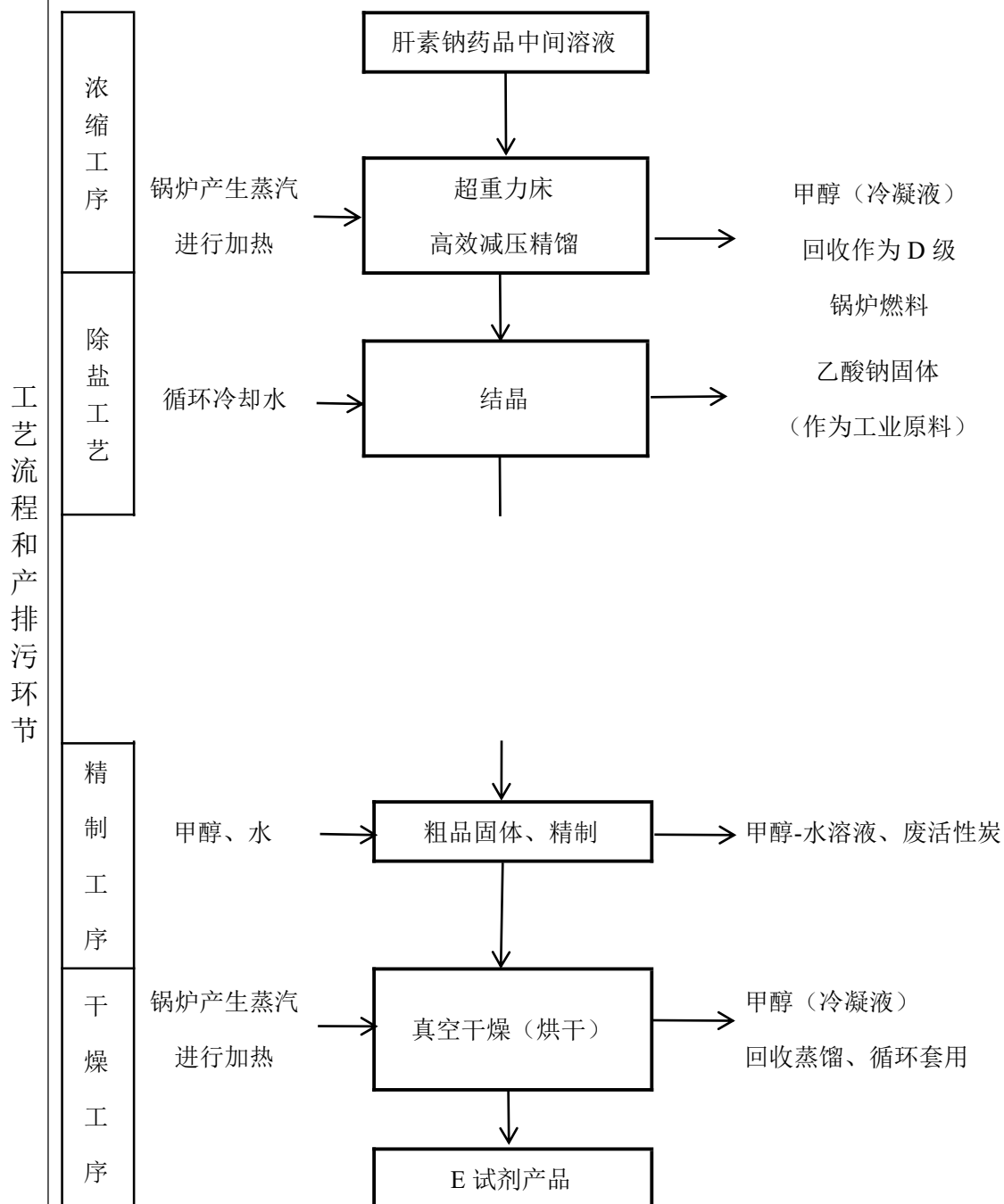
图 2-1 肝素钠药品生产用 E 试剂分离工艺流程图
