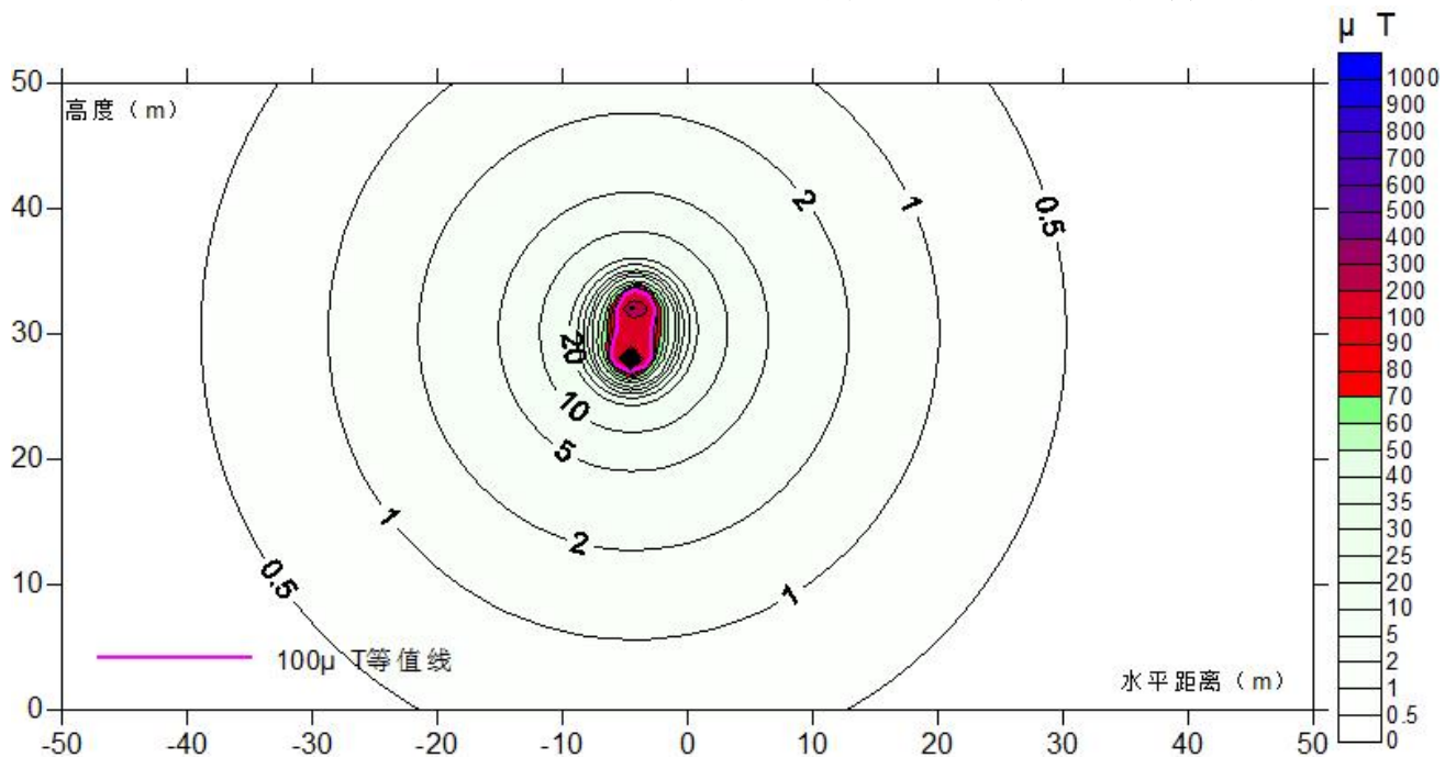
ZT-图 9.2-7 110kV 同塔双回挂单边架空线路磁感应强度预测结果等值线图
