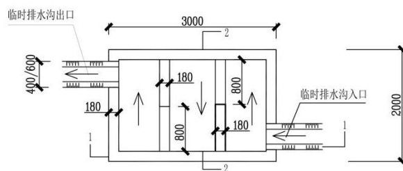
沉沙池平面图 (1: 50)
