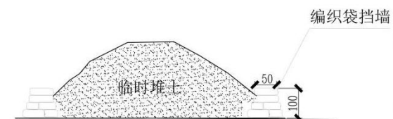
临时堆土防护设计示意图
