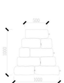
编织袋挡墙大样图 (1: 25)
