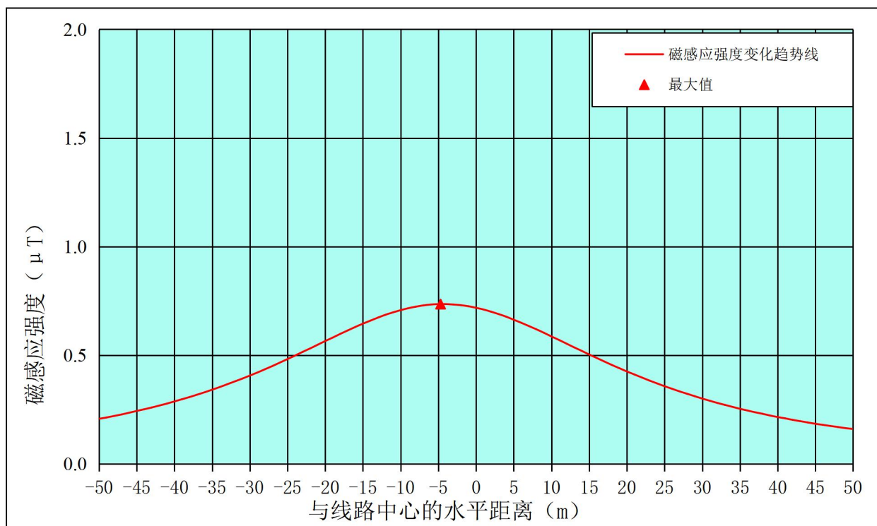
ZT-图 9.2-5 110kV 同塔双回挂单边架空线路工频磁感应强度预测结果衰减趋势线图
