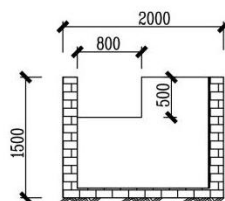
2-2剖面图 (1: 50)
