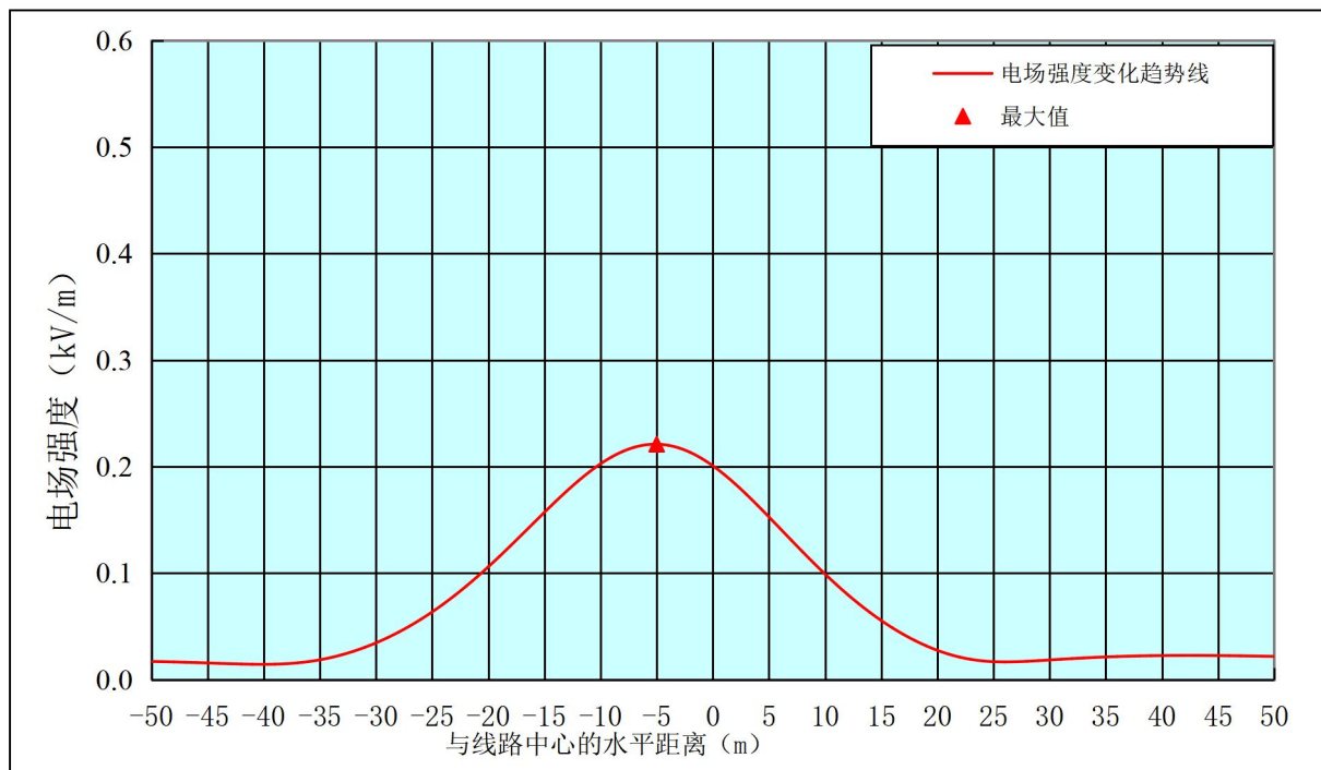
ZT-图 9.2-4 110kV 同塔双回挂单边架空线路工频电场强度预测结果衰减趋势线图
