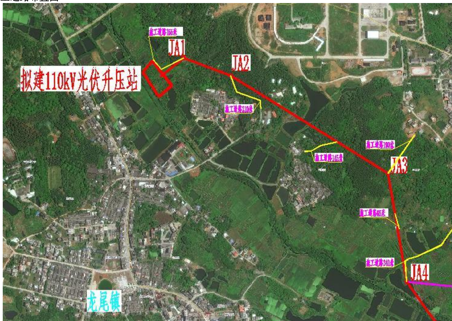
附图 13 临时施工道路布置图
