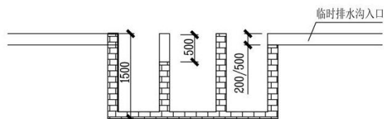
1-1剖面图 (1: 50)
