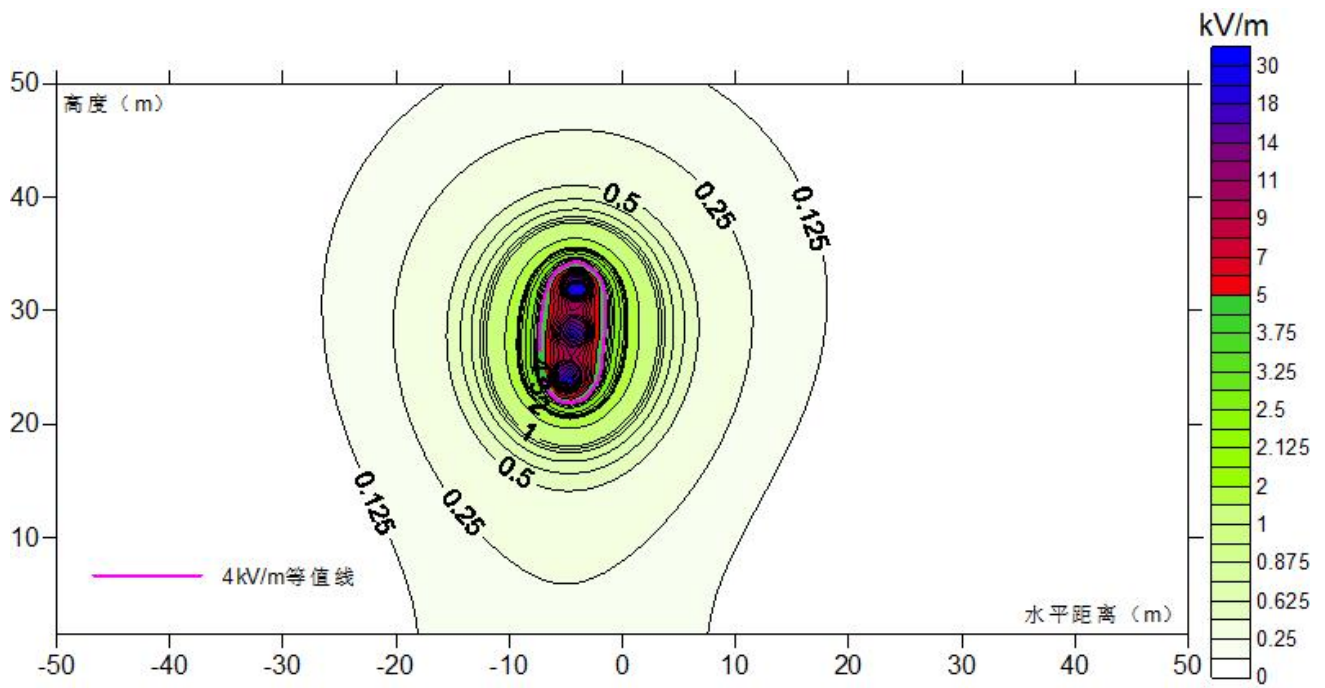
ZT-图 9.2-6 110kV 同塔双回挂单边架空线路工频电场预测结果等值线图
