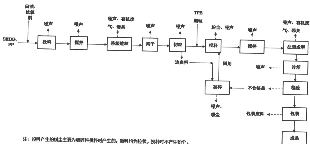
图 2-2 项目汽车垫生产线生产工艺流程图
