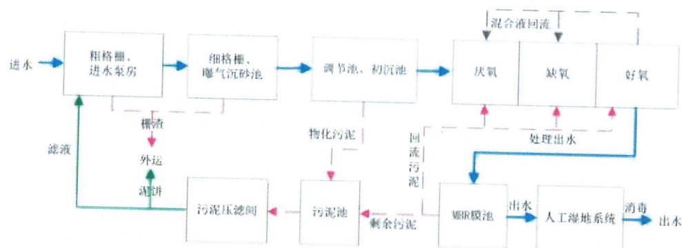
图 4.2-1 揭阳产业转移工业园东区污水处理厂生活污水工艺流程图
