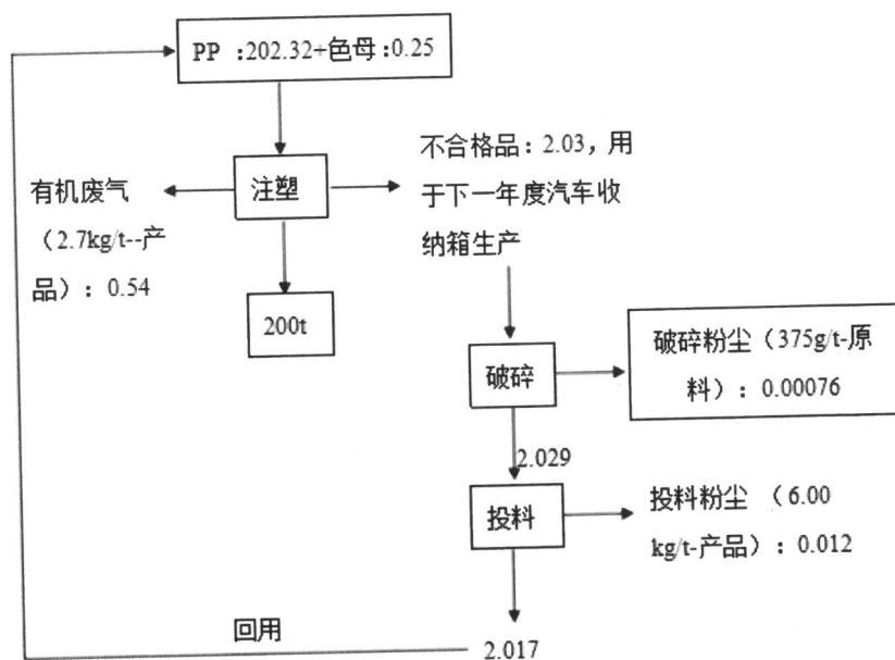
汽车收纳箱生产线物料平衡图（单位：t/a）：
