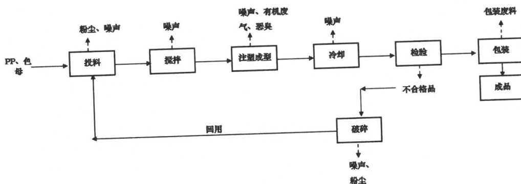
项目汽车收纳箱生产线运营期生产工艺流程图 2-3:
