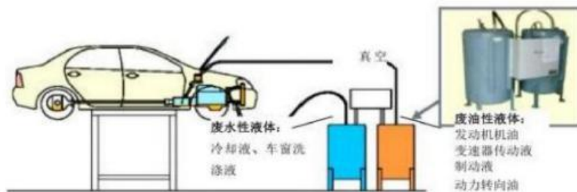
图 2-3 废液提取装置
