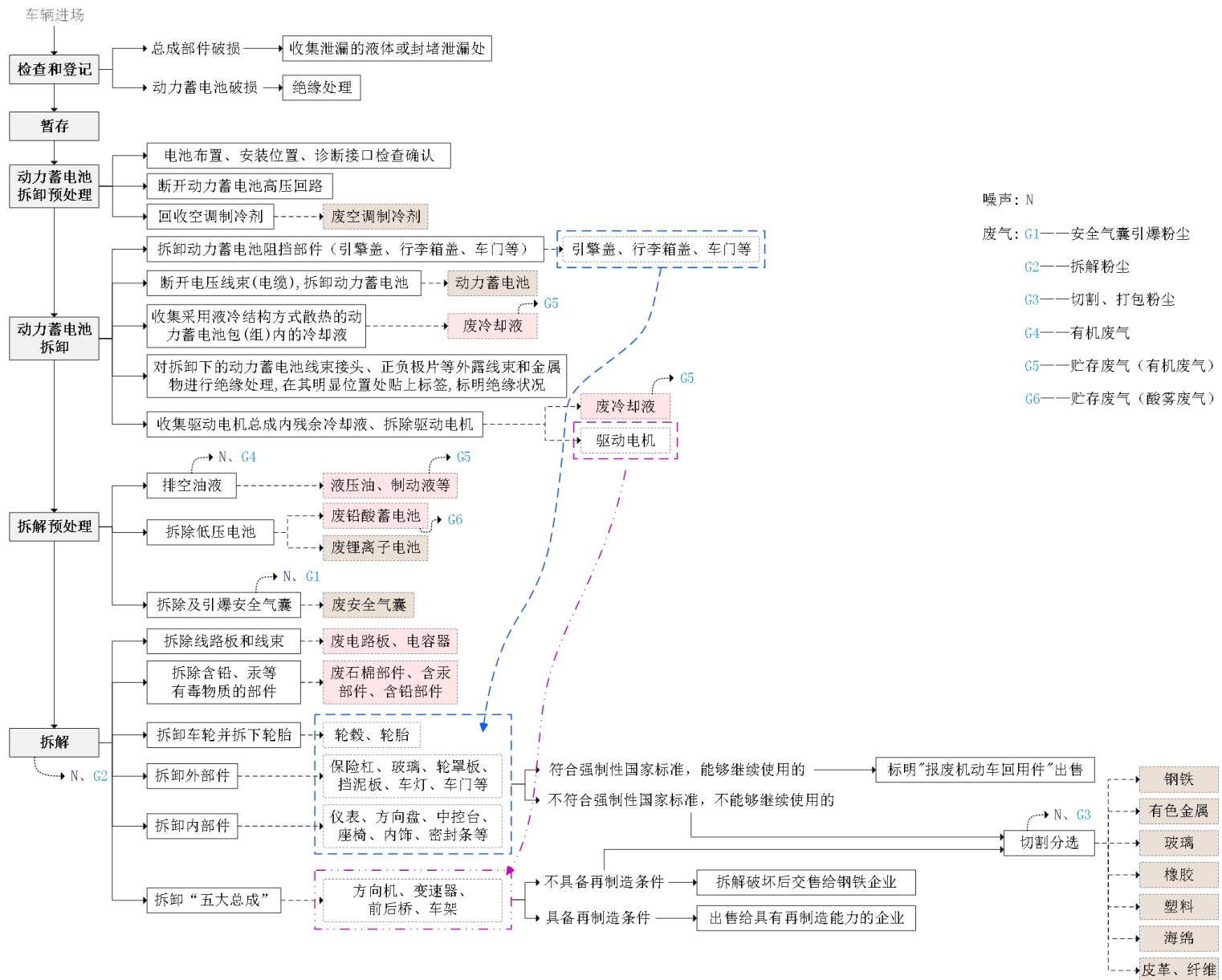
图 2-5 纯电动汽车报废拆解工艺流程
