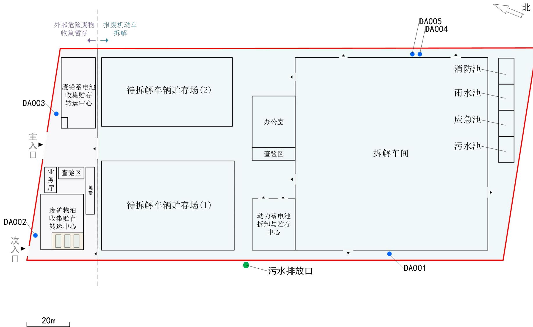
附图2 建设项目平面布置图（总平面布置）
