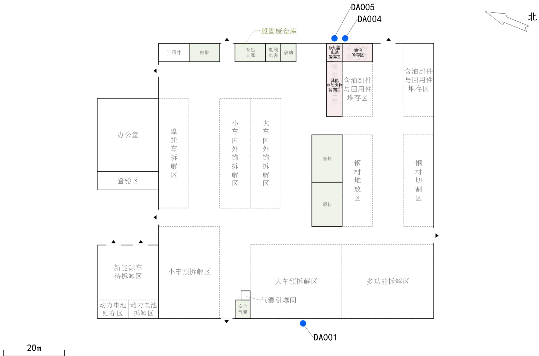
附图3 建设项目平面布置图（机动车拆解作业区）
