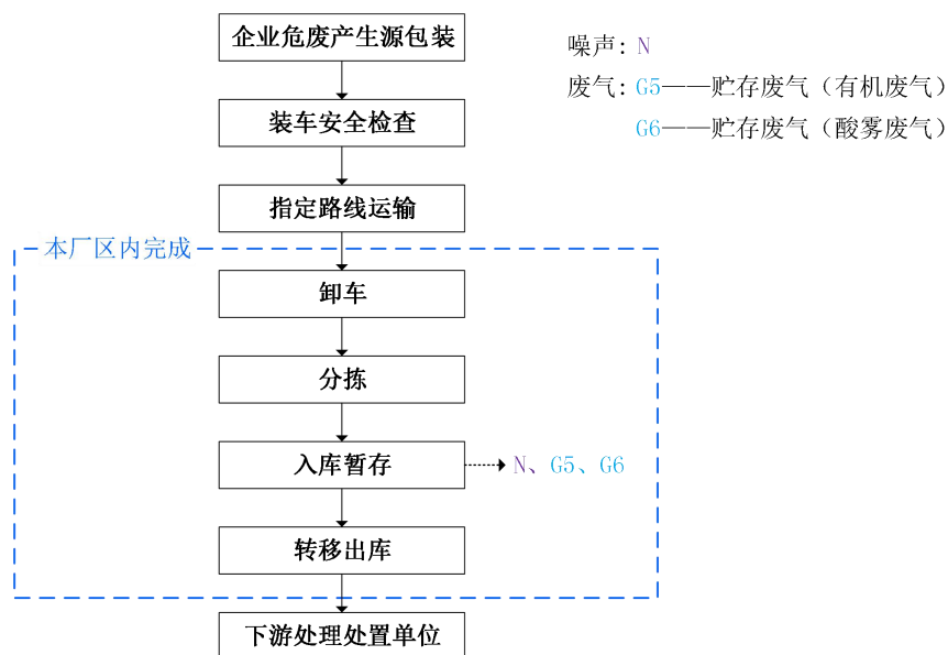
图 2-9 本项目外部危险废物收集暂存流程图
