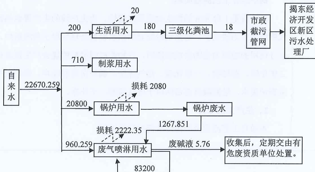
图 2-1 水平衡图 (单位: \text{m}^3/\text{a} )
