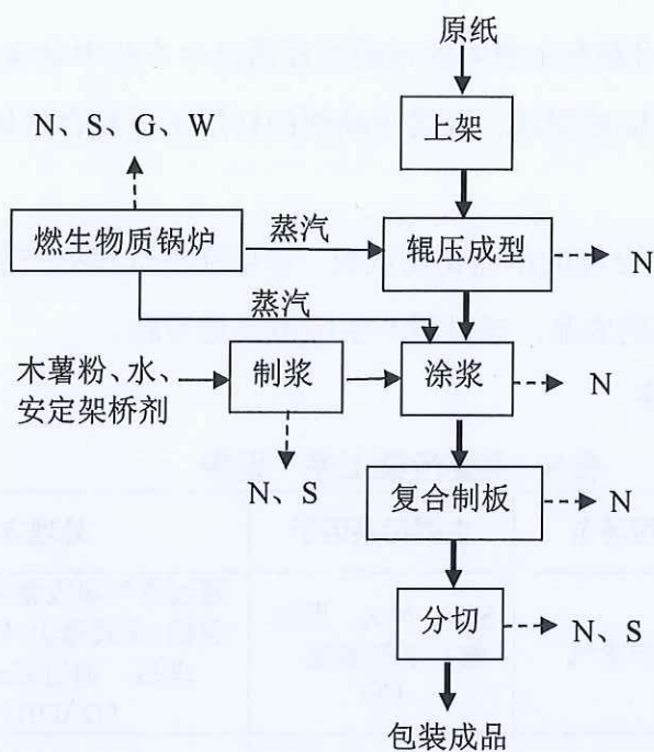
图 2-3 项目生产工艺流程图
