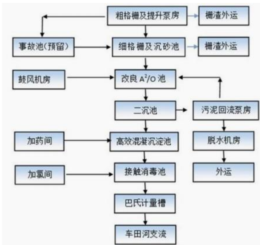
图 4-2 揭东经济开发区新区污水处理厂近期一阶段工艺流程图
