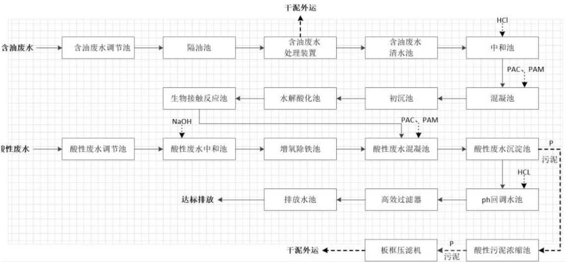
图 4-1 依托的废水处理工艺流程图
