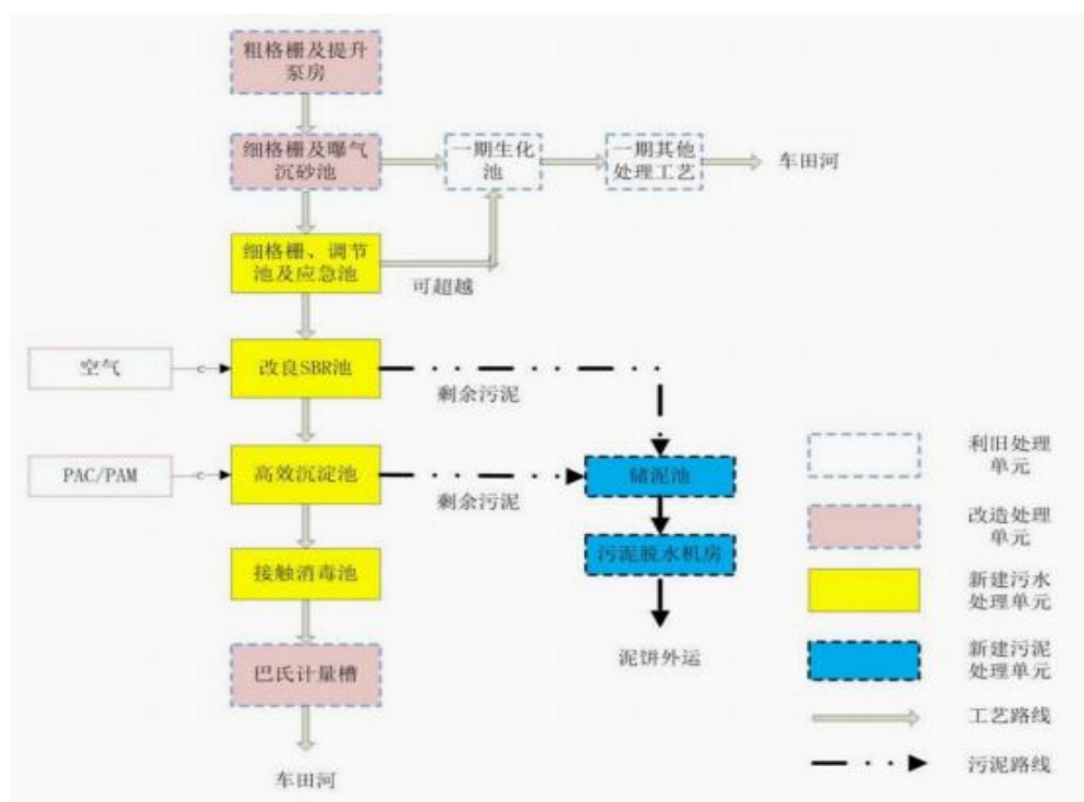
图 4-2 揭东经济开发区新区污水处理厂近期一阶段工艺流程图
