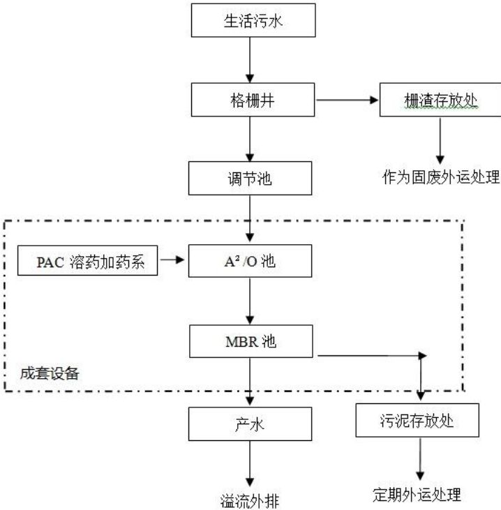
图 4-2 锡场镇锡西污水处理厂工艺流程图
