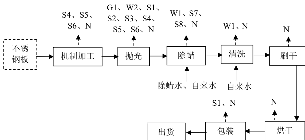
图 2-3 项目不锈钢餐厨具生产工艺流程
