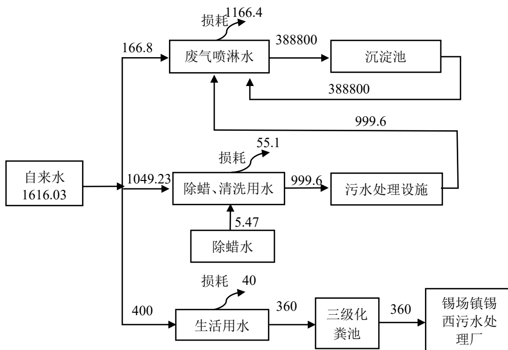
图 2-1 项目厂区水平衡图 ( \text{m}^3/\text{a} )
