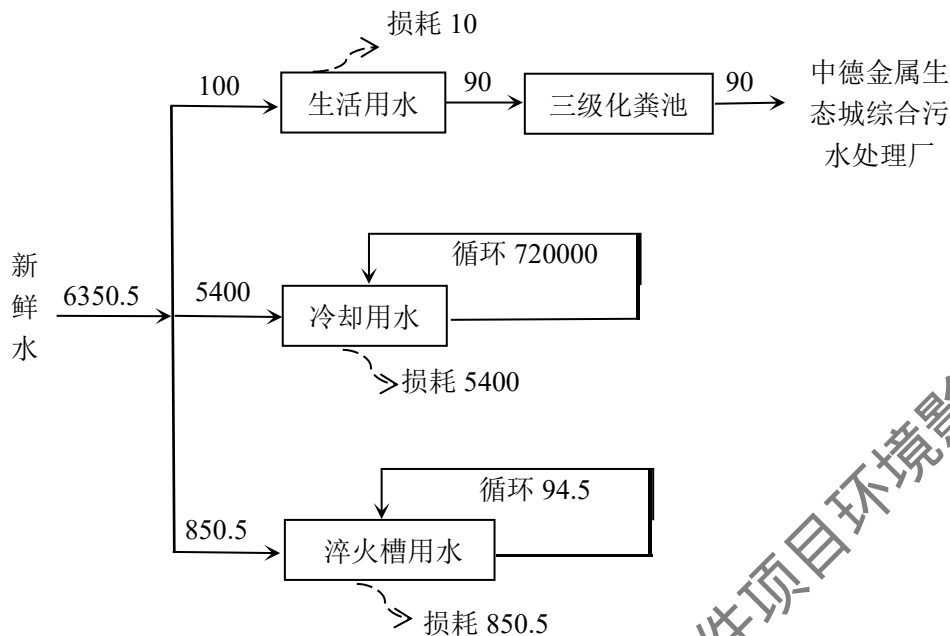
图 2-1 项目水平衡图（单位： \text{m}^3/\text{a} ）
