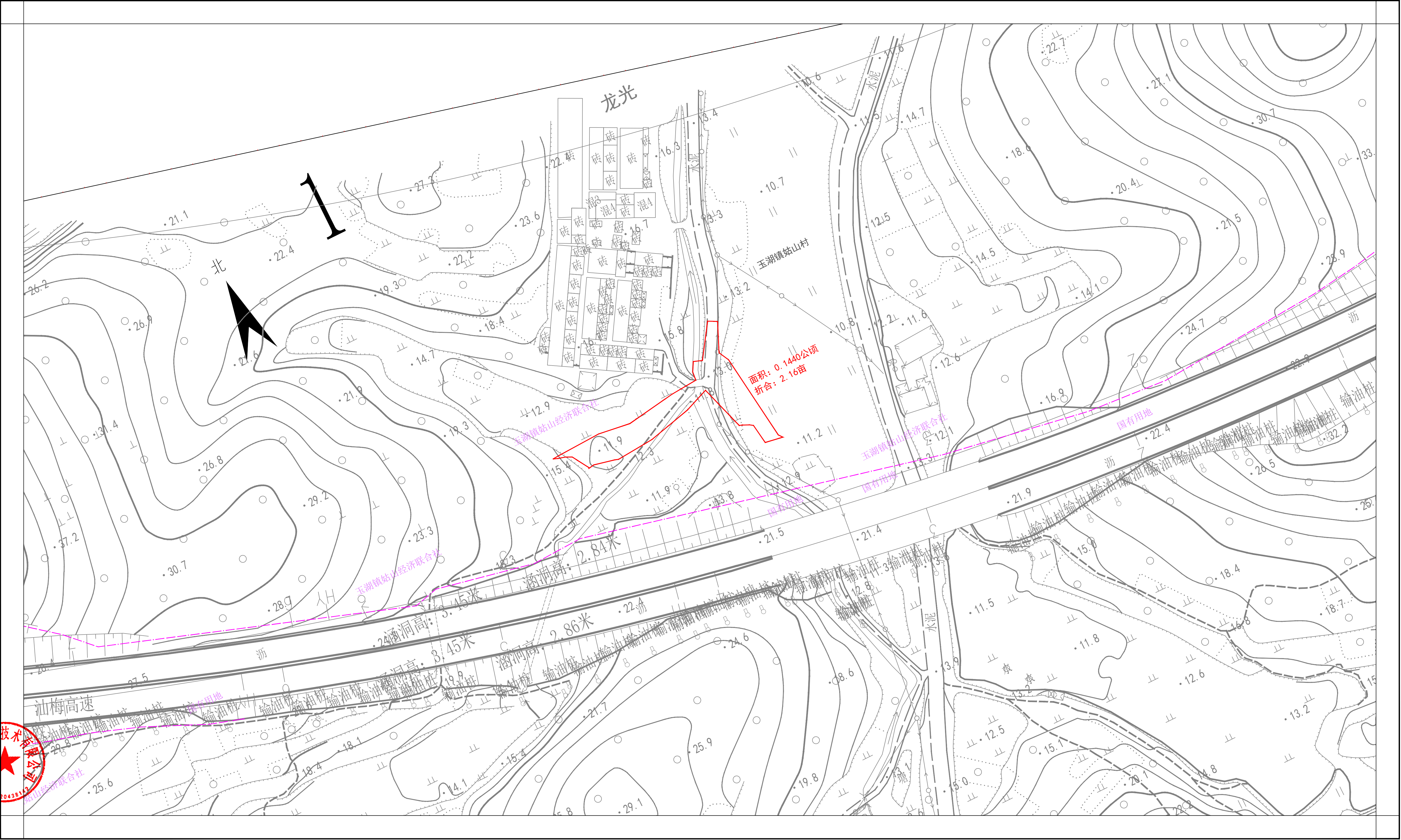
汕昆高速公路揭阳新亨至梅州畚江段及梅汕高速公路梅州程江至畚江段改扩建工程项目（揭东段）新增用地勘测定界图1 2621.7-418.3
