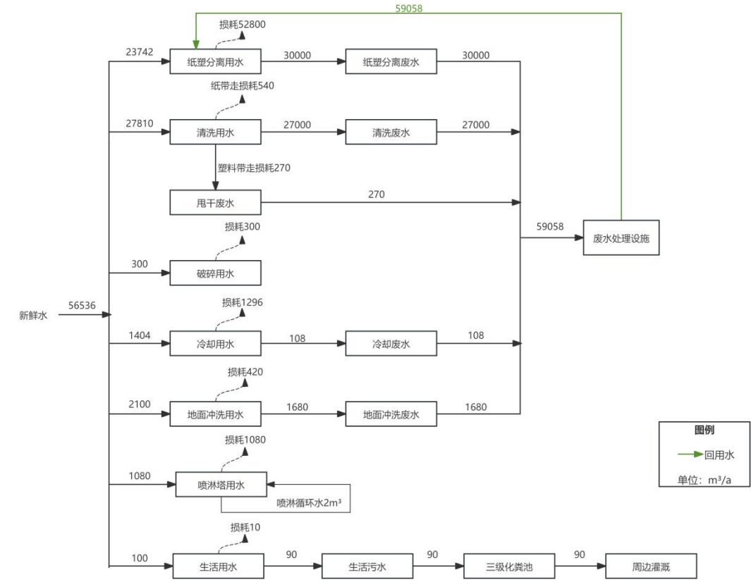
图 4.2-1 水平衡图
